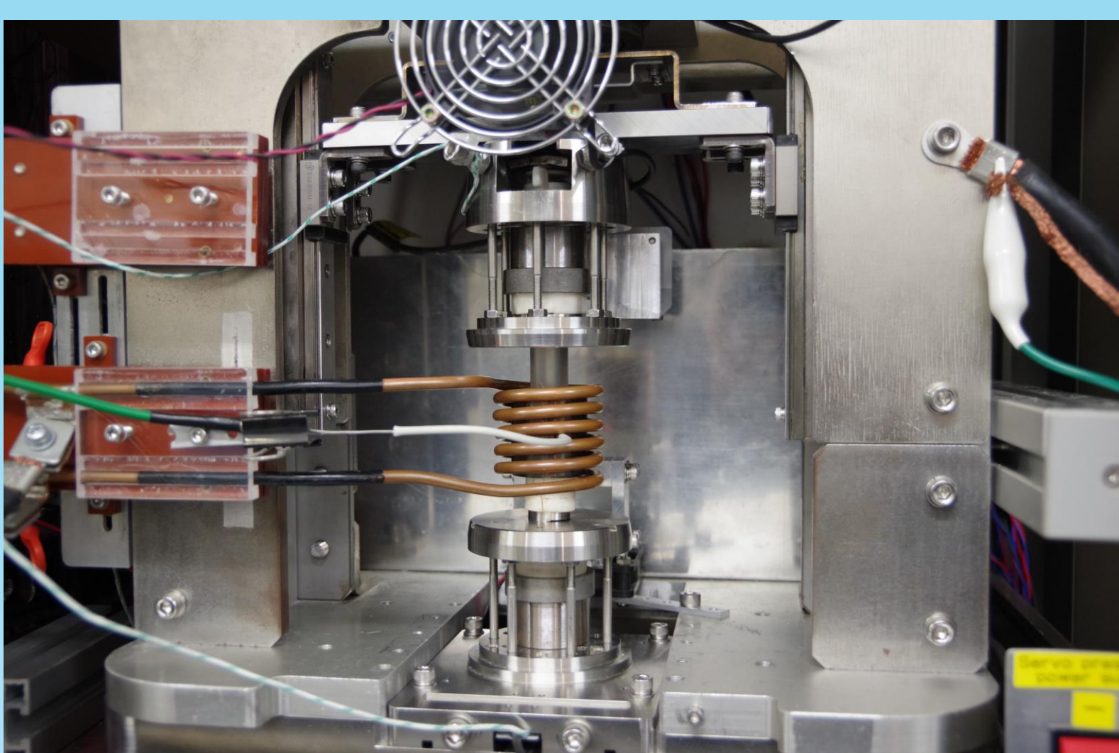
測定状態
