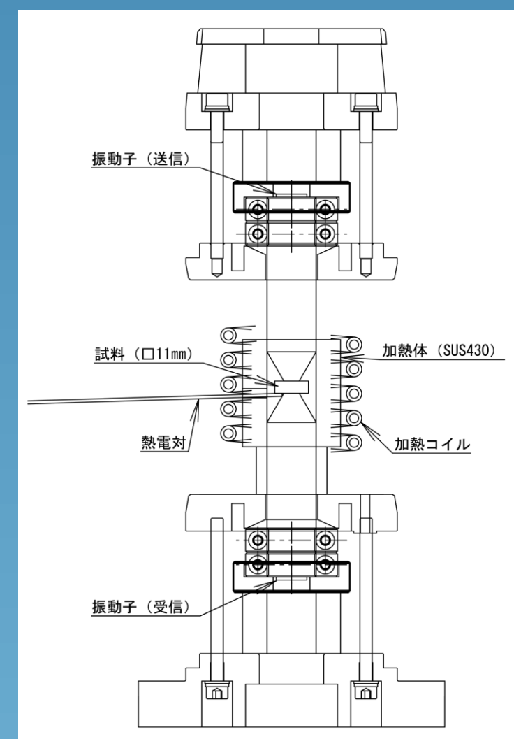
測定状態図
