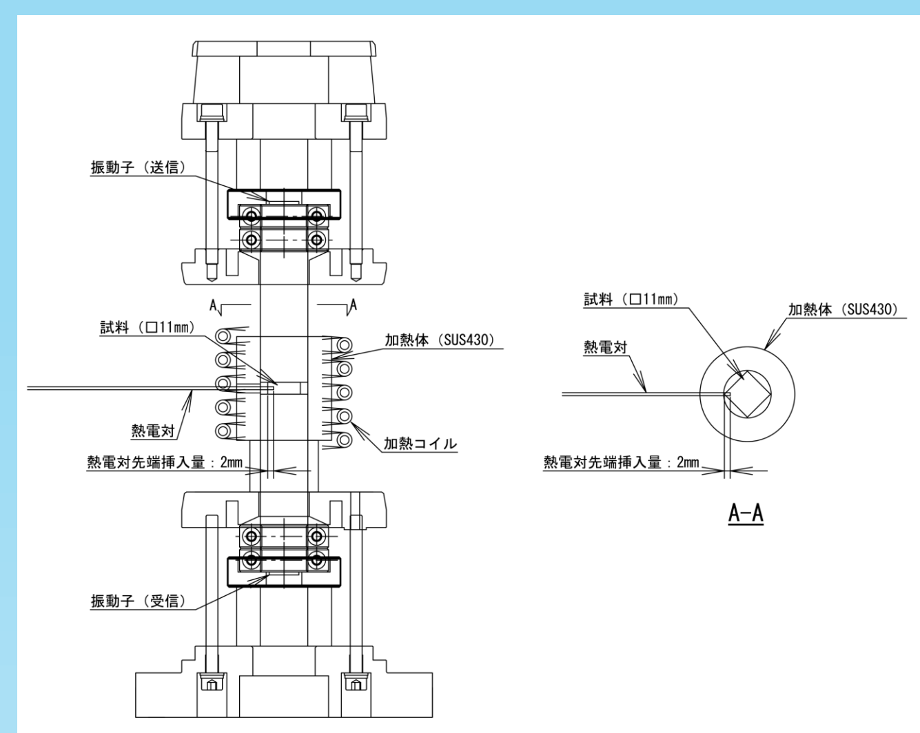
測定状態図
