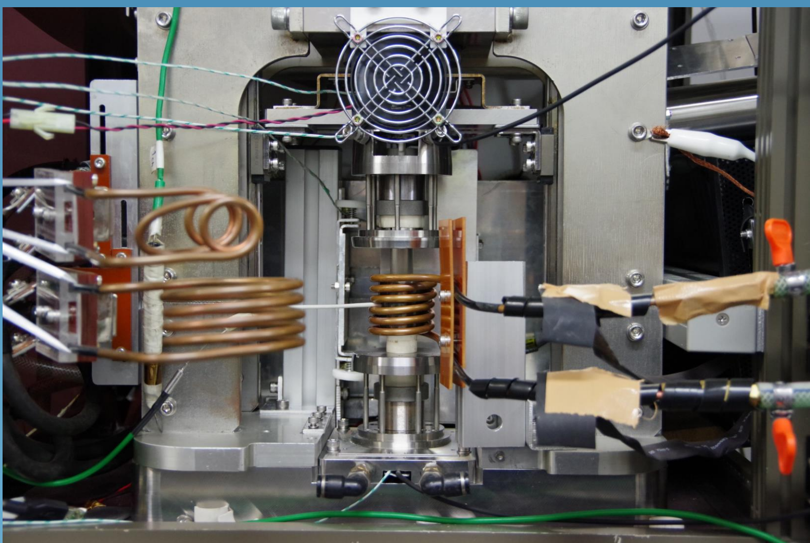
測定状態
