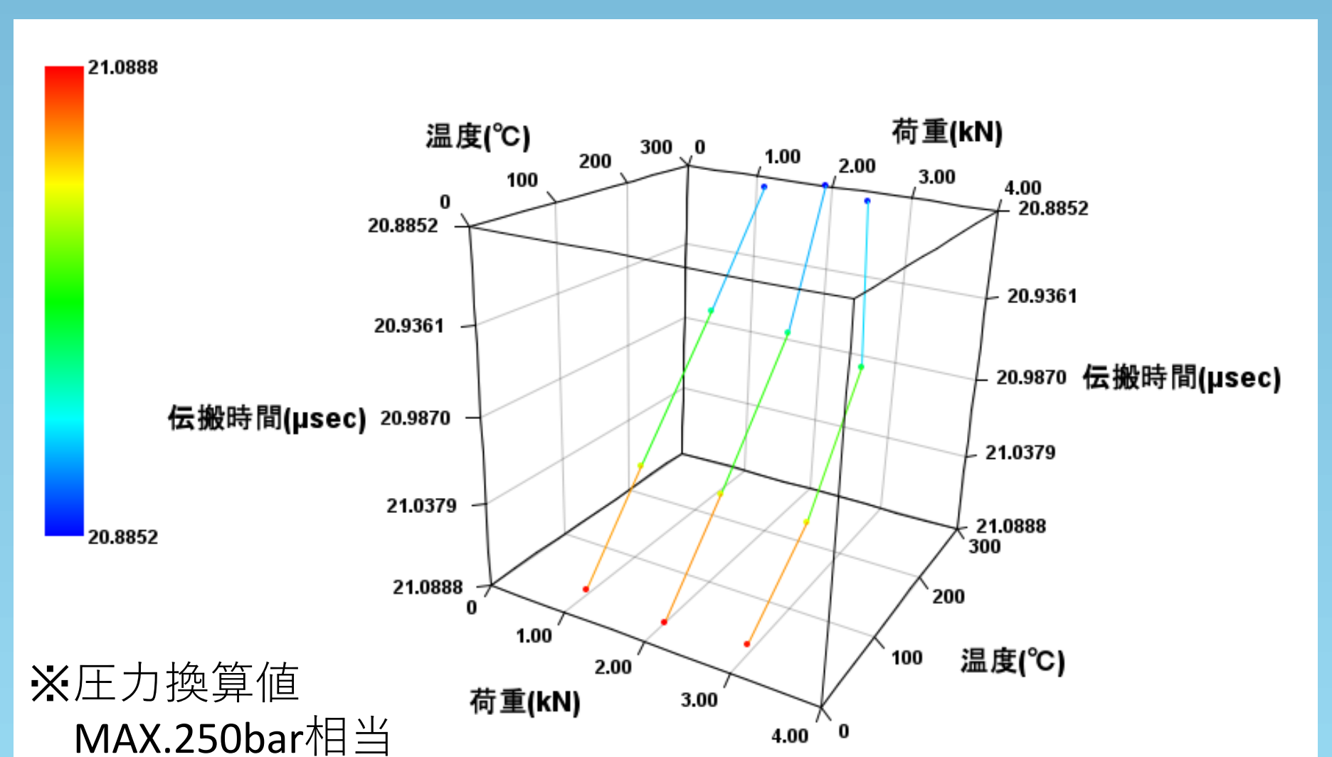
計測結果
