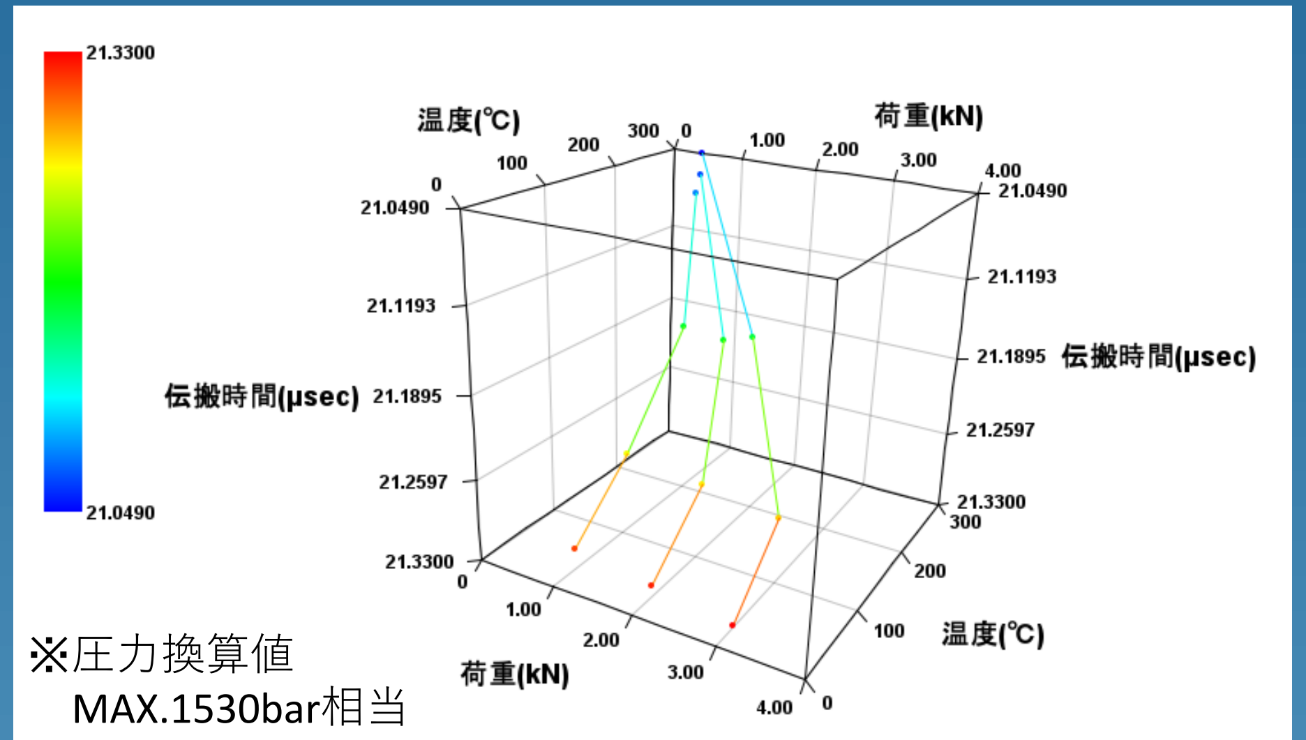
計測結果
